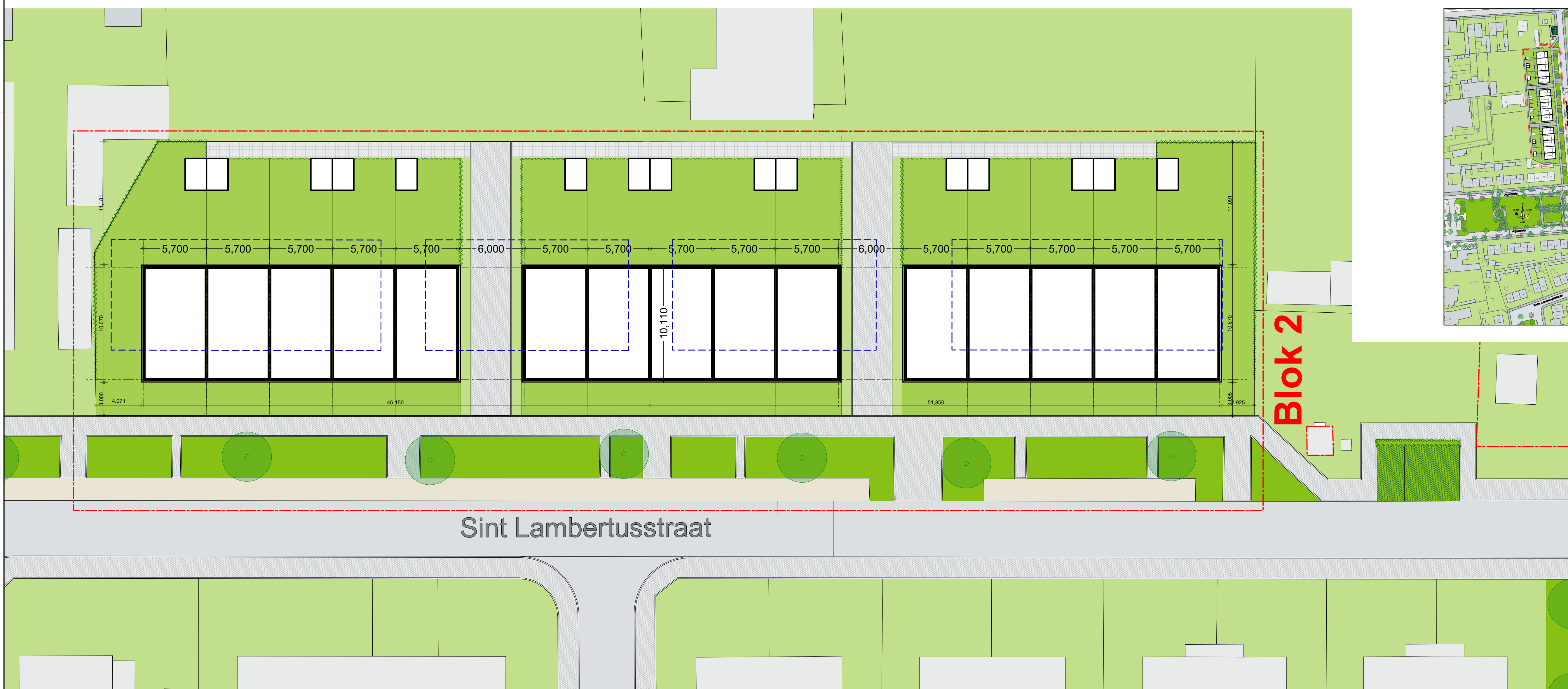
Blok 2 Situatie Nieuw 1:200
