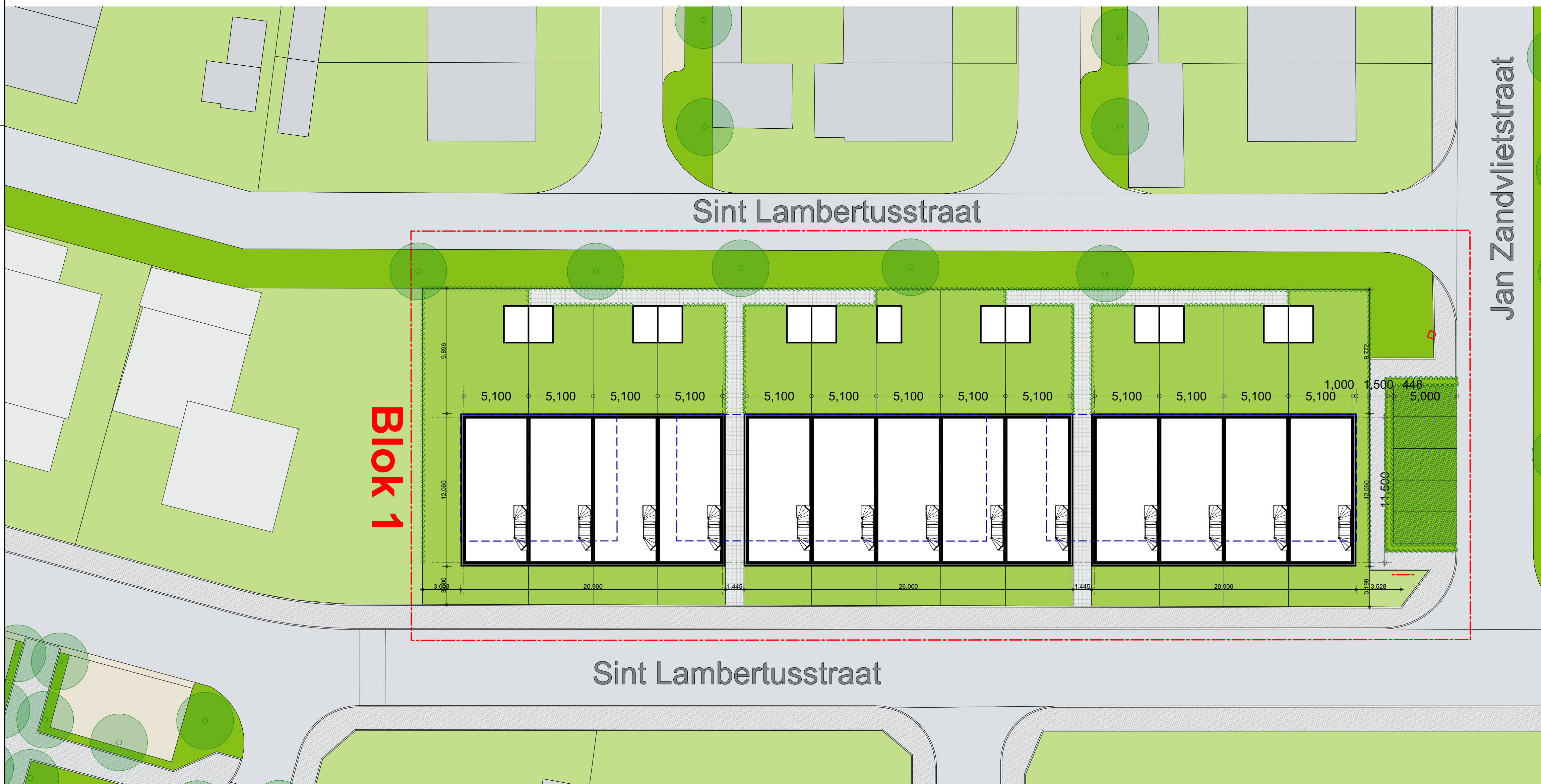
Blok 1 Situatie Nieuw 1:200
